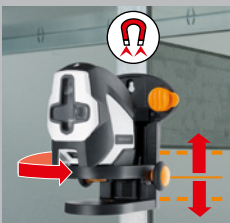
Trípode/soporte de pared regulable en altura
